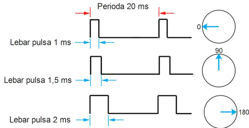
Gambar 4. Kontrol PWM pada pergerakan motor
