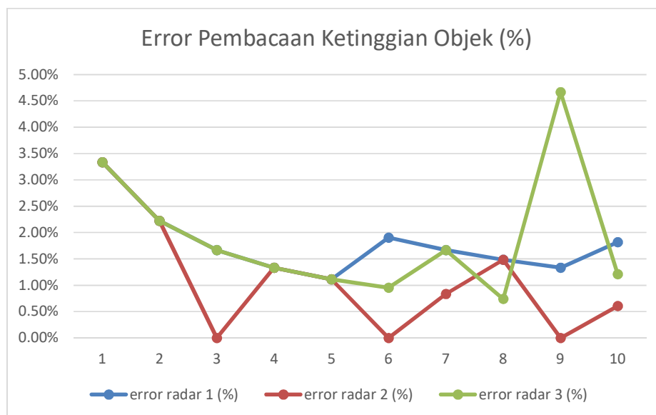
Gambar 11. Nilai kesalahan pembacaan ketinggian
