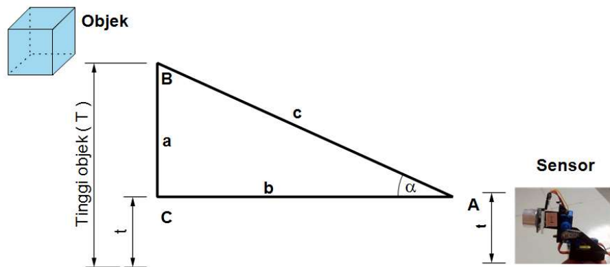
Gambar 6. Kalibrasi ketinggian penempatan sensor
