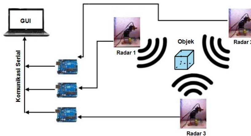
Gambar 7. GUI aplikasi dan penempatan sensor radar
