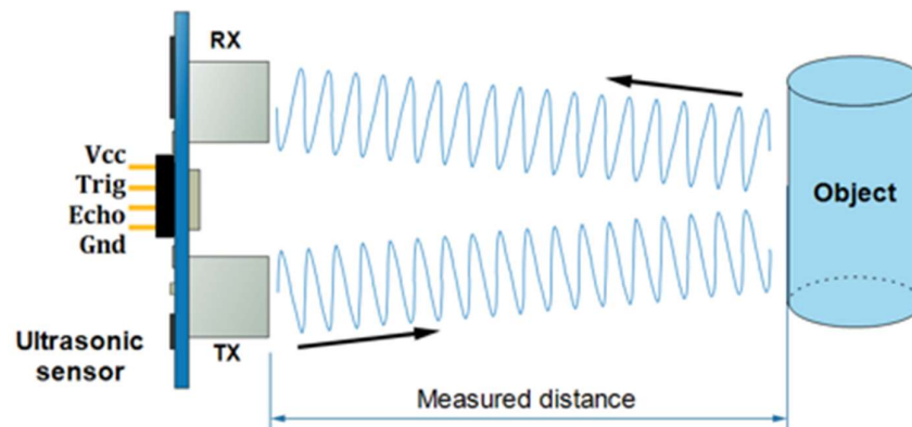
Gambar 1. Cara kerja sensor ultrasonik
