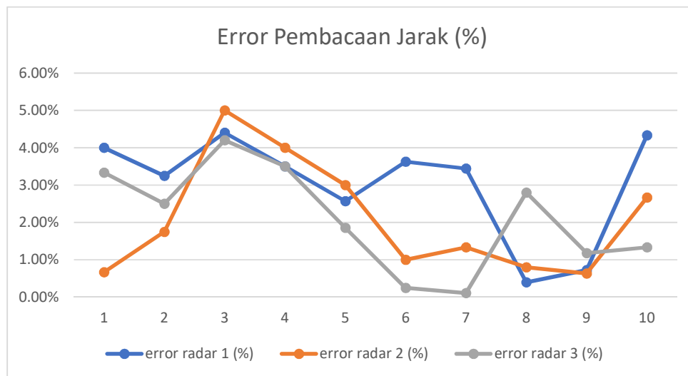
Gambar 10. Nilai kesalahan pembacaan jarak
