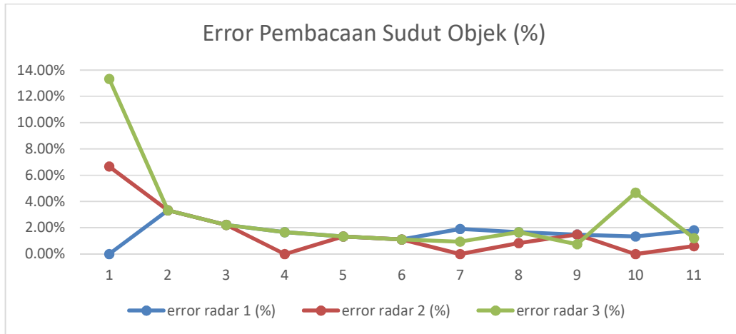
Gambar 12. Nilai kesalahan pembacaan sudut
